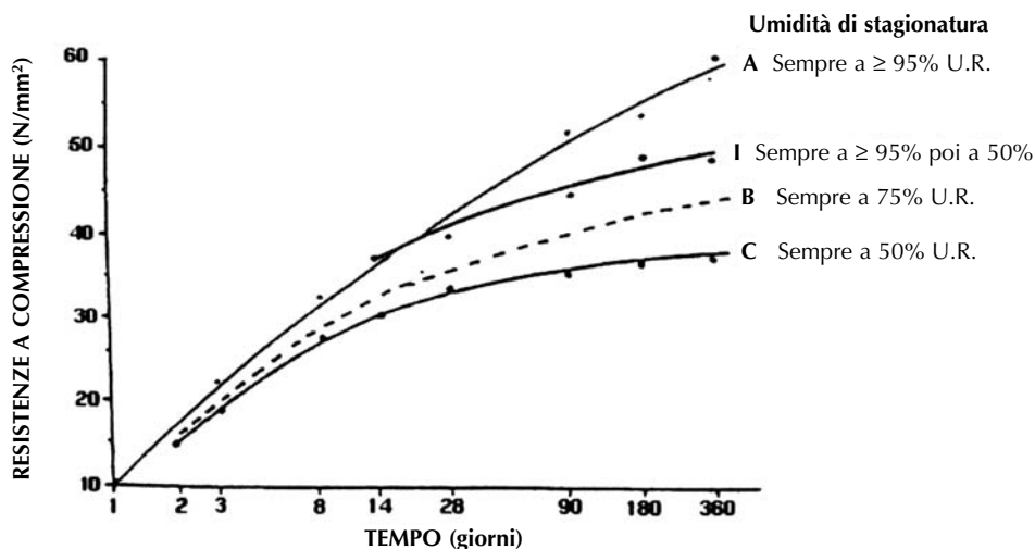
Figura 6 - Effetto di diverse condizioni igrometriche di stagionatura sullo sviluppo delle resistenze del calcestruzzo; provino di 10 cm di lato (CNR, Boll. Ufficiale 23.12.92, parte IV - Norme Tecniche).
