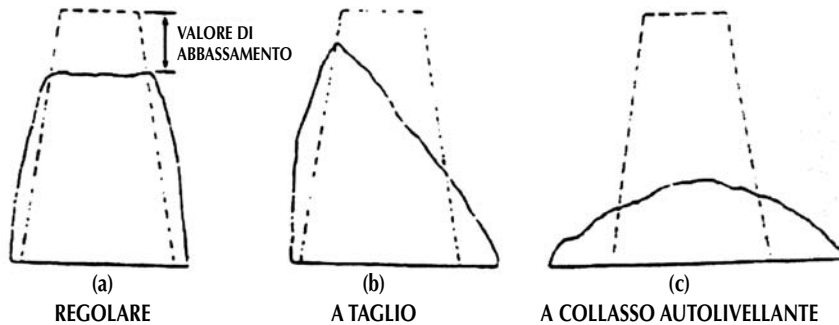
Figura 1- Forme di abbassamento al cono.
