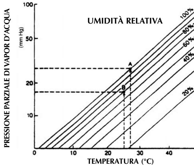
Figura 3 - Pressione parziale del vapore acqueo in funzione della temperatura.
