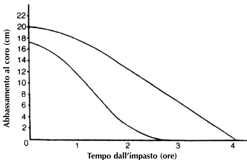
Figura 2 - Andamento della diminuzione di lavorabilità degli impasti di calcestruzzo.
