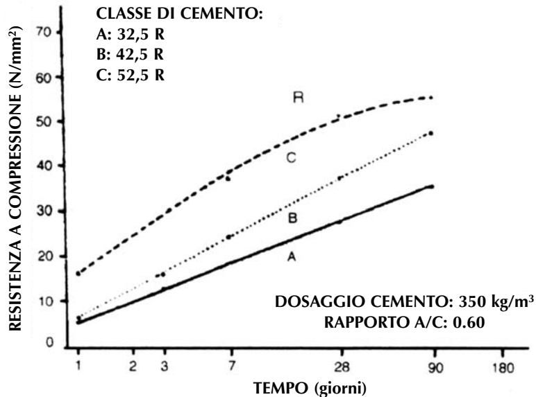
Figura 5 - Esempio di sviluppo della resistenza a compressione di calcestruzzi di pari composizione in relazione a tre classi di cemento (CNR, Boll. Ufficiale 23.12.92, parte IV - Norme Tecniche).
