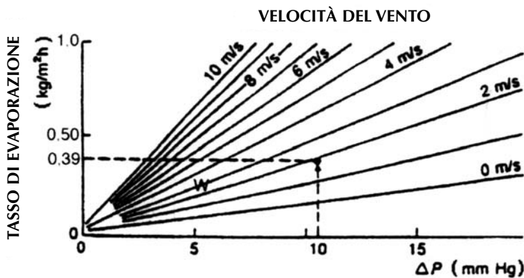
Figura 4 - Velocità di evaporazione in funzione della velocità del vento e della pressione parziale del vapore.
