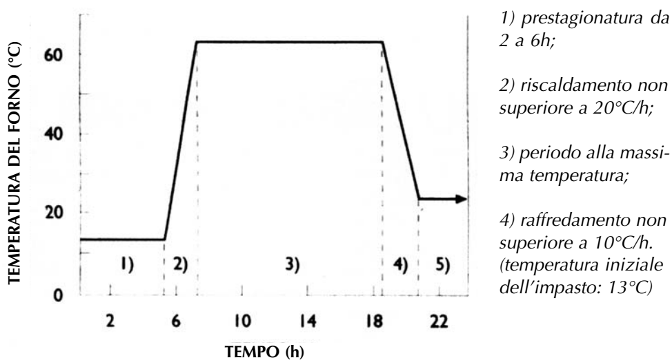
Figura 7 - Esempio di stagionatura a vapore alla pressione ordinaria.
