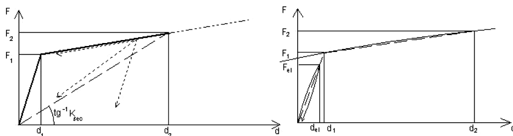
Figura 9.1 - Diagrammi forza-spostamento per dispositivi a comportamento non lineare
