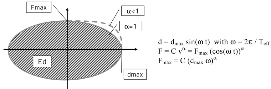
Figura 9.2 – Dispositivi a comportamento viscoso
